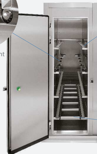
Aménagement à rouleaux Tubular beam with full width rollers
